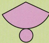
Cone
